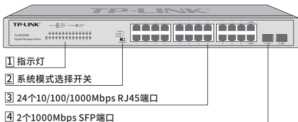
图1-3 TL-SG2226前面板示意图
